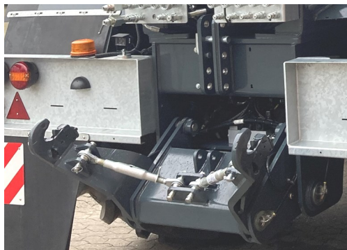
Lift med 8 ton løfte kapacitet, monteret så redskabet sidder tæt på vognen.
