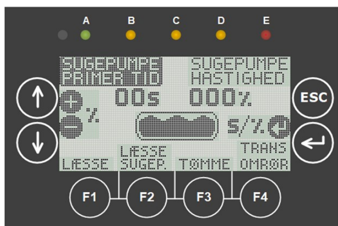
Skærbillede under normal drift, her indstilles primer tid og hastighed.
