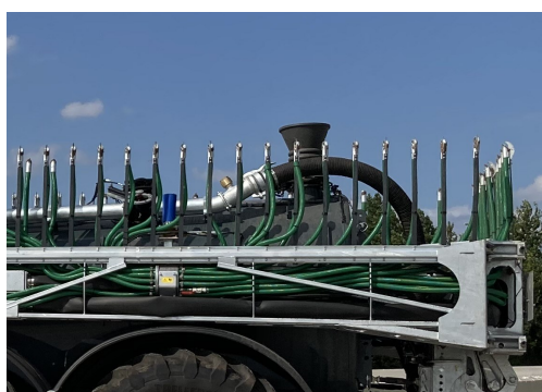
Ekstern fyldetragt 10", rotorblink giver signal ved fuldtank.
