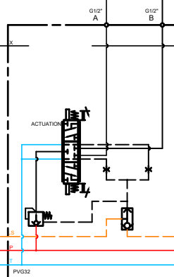
Doseringsventil M0 C1 P42 X4.13
