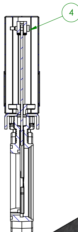
SECTION A-A
